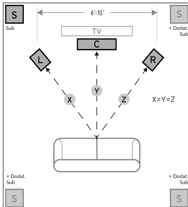
Rysunek 1 Rozstawienie głośników w miejscu odstuchu
