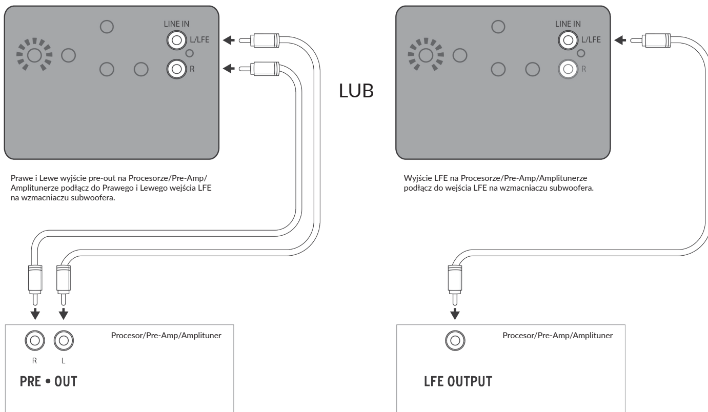
Rysunek 2 Wejścia liniowe
